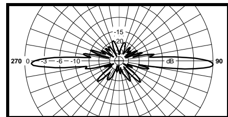
E-Plane
